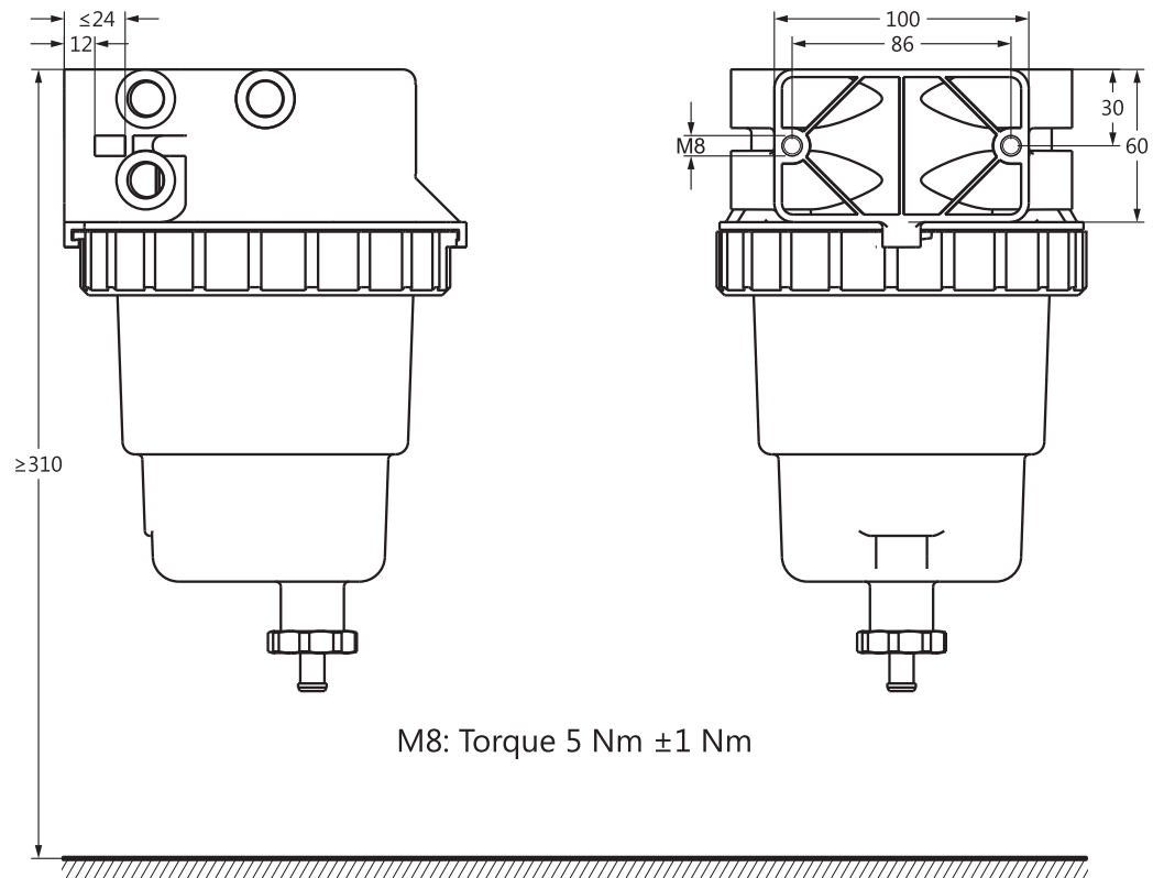
Abbildung 6: Montagemaße
